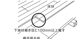
ネダレス工法(構造用合板捨貼りの場合)
