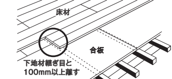
在来工法(合板捨貼りの場合)
